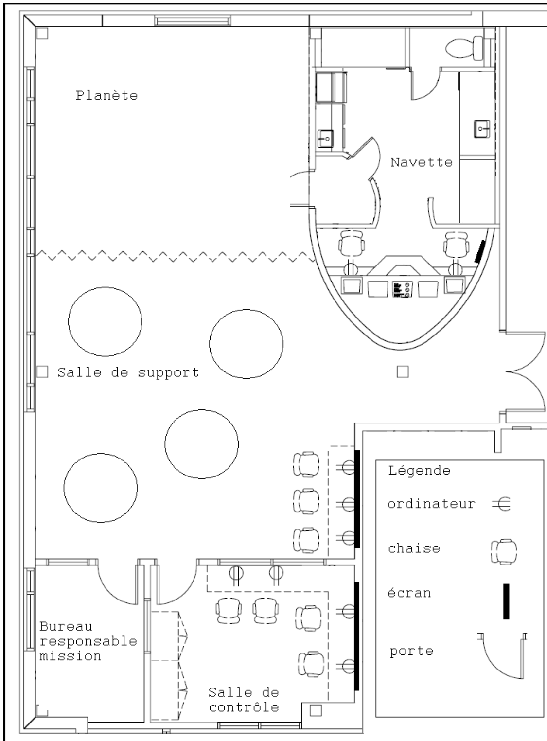
Plan du Centre de simulation en science et technologie (CENST)
